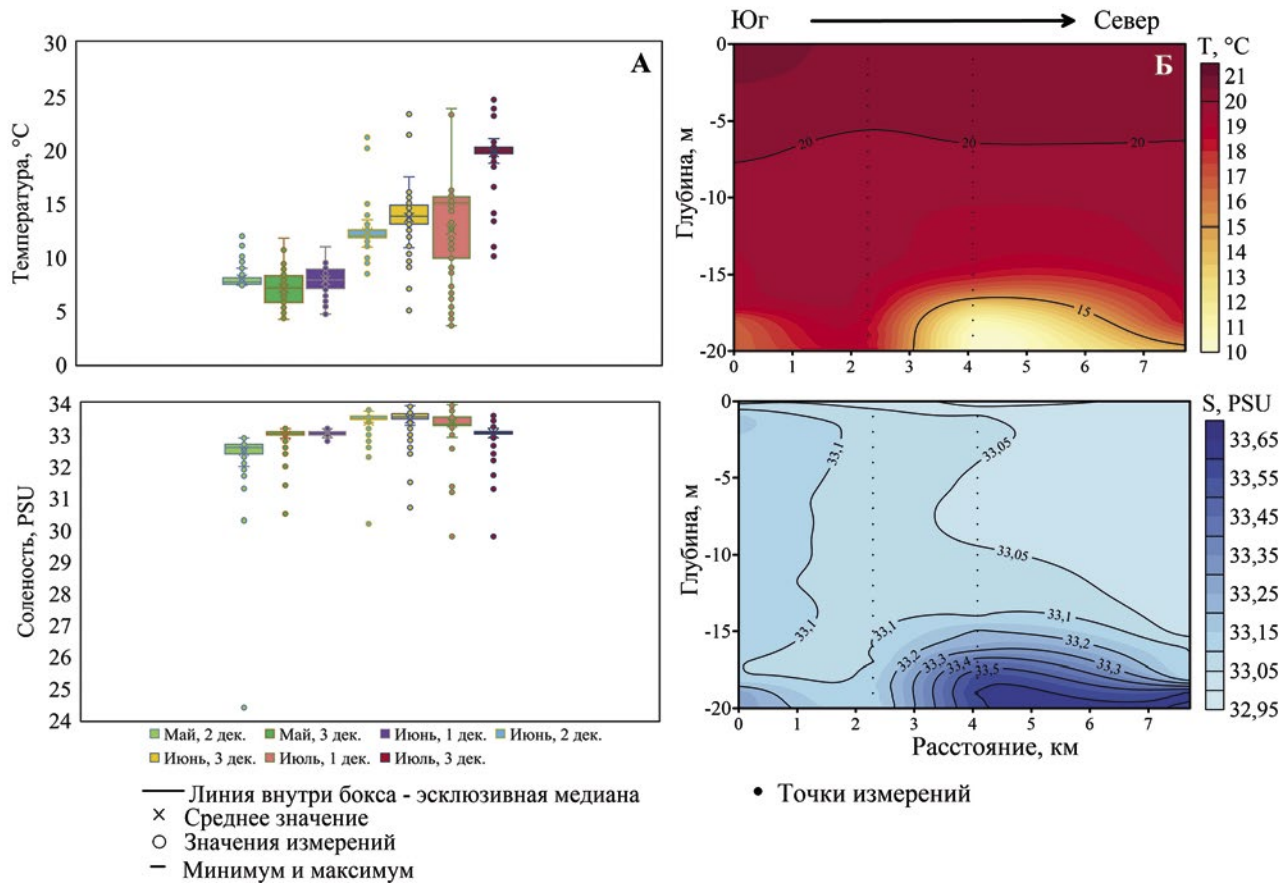
Рис. 2. Сезонные изменения температуры и солености воды в юго-восточной части Татарского пролива в 2025 г (А), вертикальный профиль температуры и солености в третьей декаде июля на глубине 20 м (Б)
