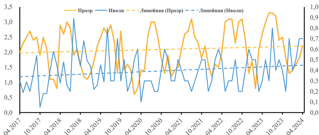
Рис. 6. Среднемесячная высота волн (H волн, м) – правая ось и прозрачность воды (Прозр, м) – левая ось в 2017-2024 гг.
