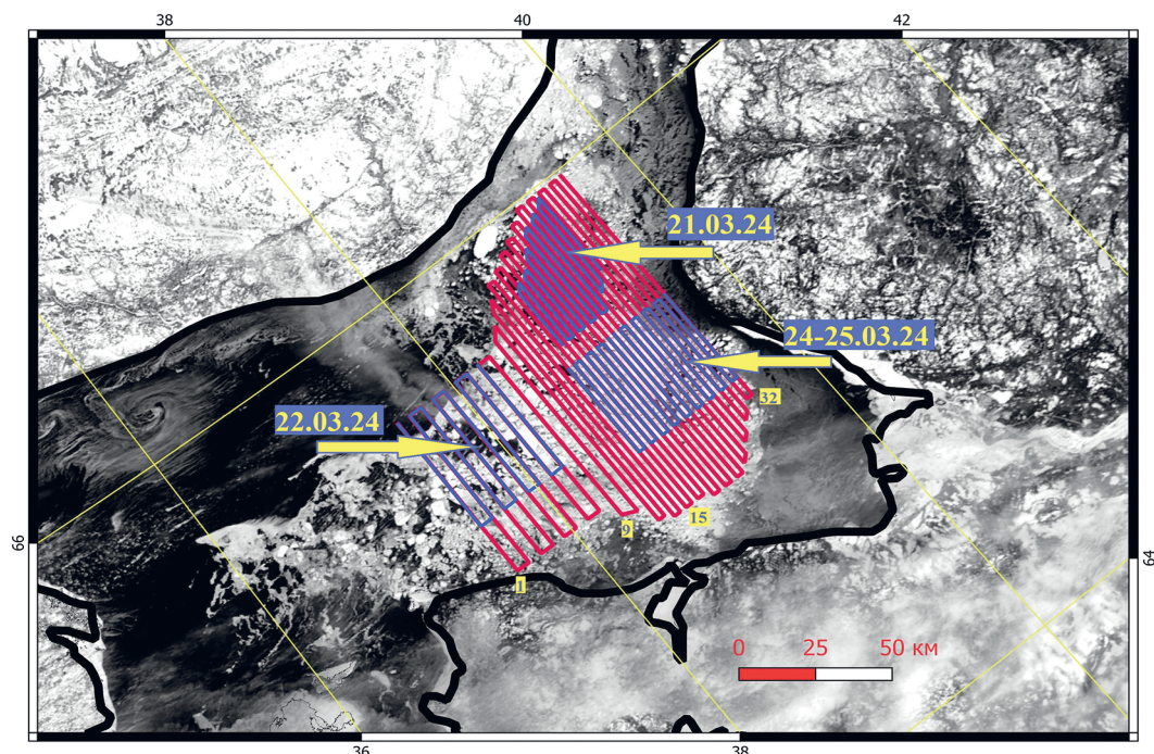
Рис. 8. Карта схема расчётной области ледового массива в Бассейне Белого моря. Красные полосы – расчётная область из 32 линий, пронумерованных с запада на восток, стрелками показаны синие полосы – трансекты авиаучётов с 21 по 25 марта 2024 г.
