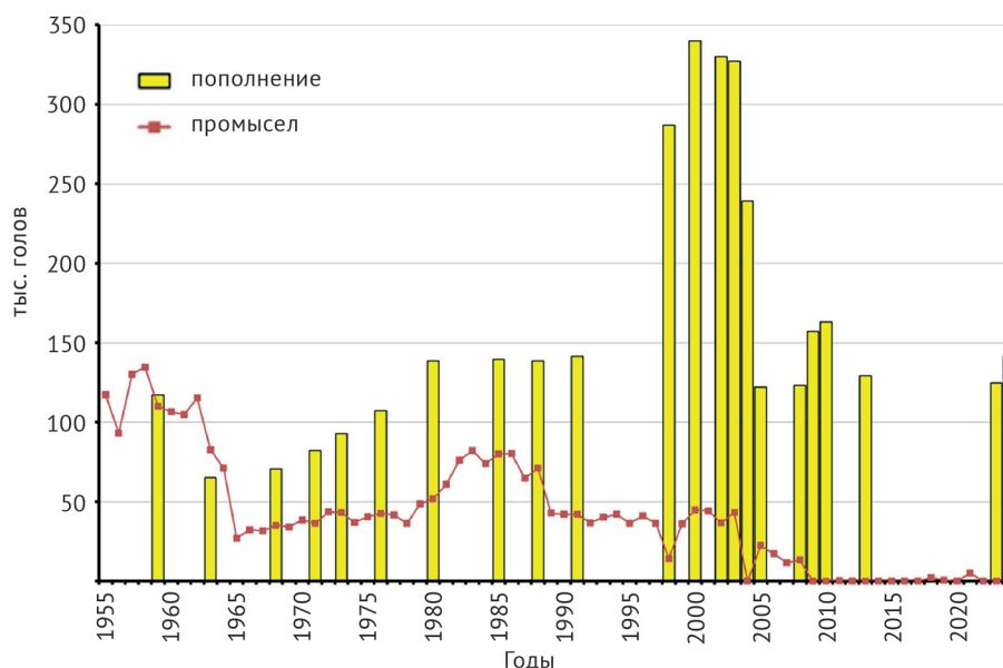
Рис. 12. Изменение численности пополнения по данным авиасъёмок и динамика промысла ГТБП с 1955 по 2024 гг. [по данным: Назаренко, 1984; Черноок и др., 1999; Шафилов, 2015; ICES. 2023; собственные данные]
