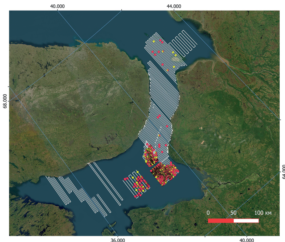
Рис. 7. Распределение щенков и половозрелых особей на дрейфующих льдах Белого моря с 3 по 25 марта 2024 г. Fig. 7. Distribution of pups and adults on drift ice of the White Sea from March 3 to March 25, 2024
