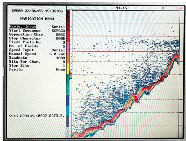
Рис. 8. Эхограмма пелагических скоплений омуля. Диапазон глубин от 235 до 80 м
