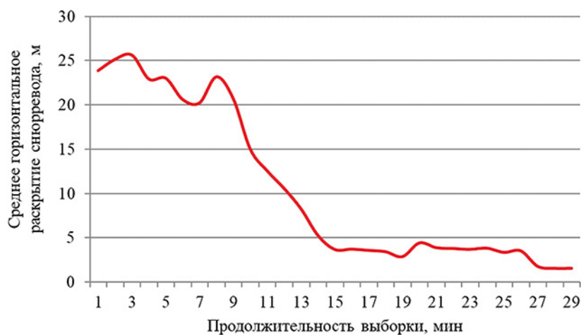
Рис. 9. Изменение горизонтального раскрытия снурревода в процессе выборки урезов ( n_{\text{замётов}} = 46 )
