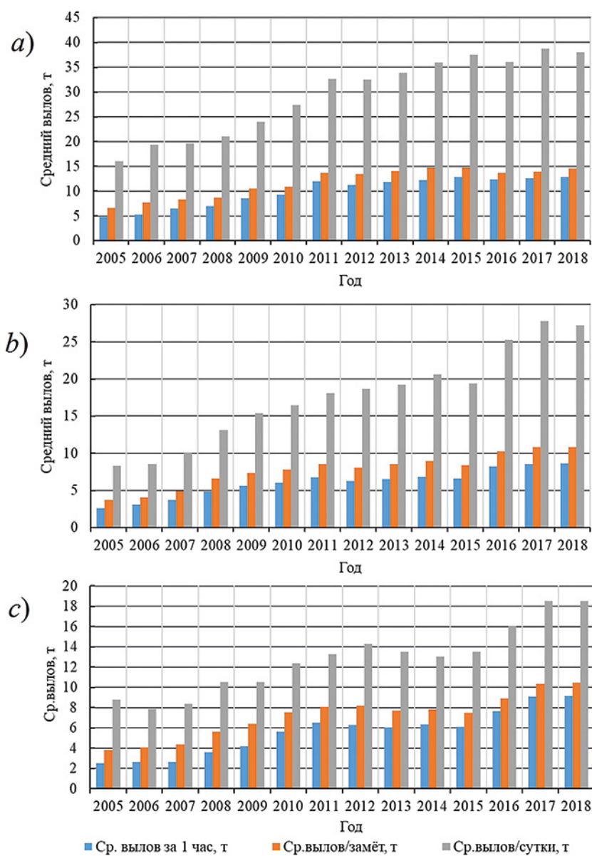
Рис. 17. Параметры интенсивности лова по классу судна в период 2005–2018 гг. а – средние суда, б – малые суда, с – малые маломерные суда
