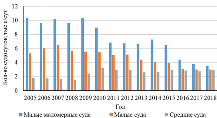
Рис. 15. Количество судо-суток, отработанных флотом на снюрреводном лове в период 2005–2018 гг.
