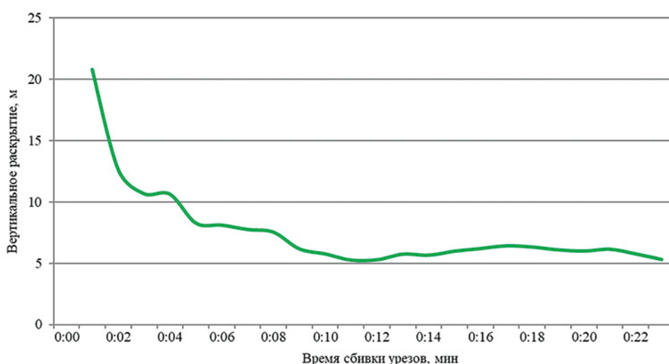
Рис. 10. Изменение вертикального раскрытия снурревода во время сбивки урезом ( n_{\text{замётов}} = 46 )
