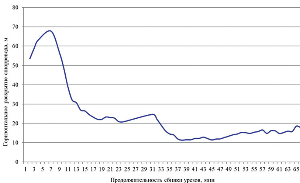
Рис. 8. Горизонтальное раскрытие снюрревода в процессе сбивки урезков с увеличенной продолжительностью
