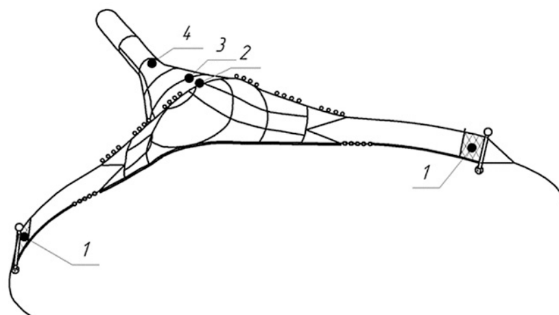
Рис. 2. Схема установки датчиков гидроакустического комплекса «ScanMar» на снюрреводе датского типа: 1 – датчики расстояния; 2 – траловый зонд; 3 – датчик глубины; 4 – датчик температуры
